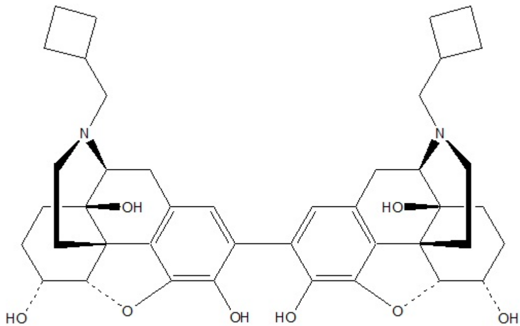
Bis-nalbuphine
